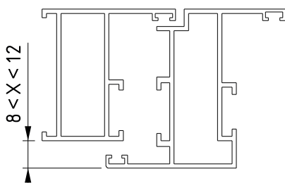
Profilabmessung
